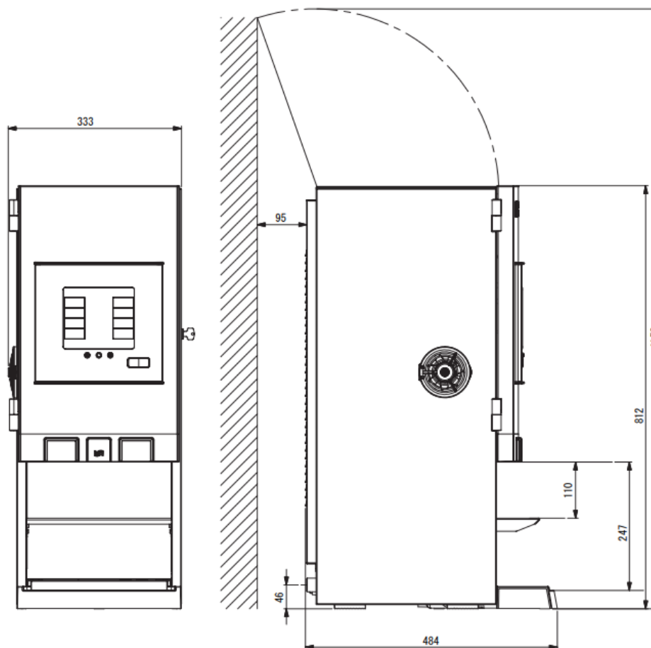
Zijaanzicht (met deksel open)
